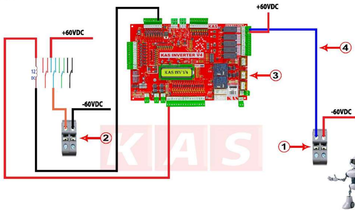
مخطط توصيل عدد 2 باب فولدينج Connection diagram of 2 folding doors
