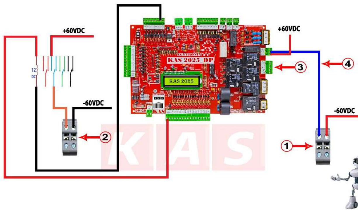
مخطط توصيل عدد 2 باب فولدينج Connection diagram of 2 folding doors
